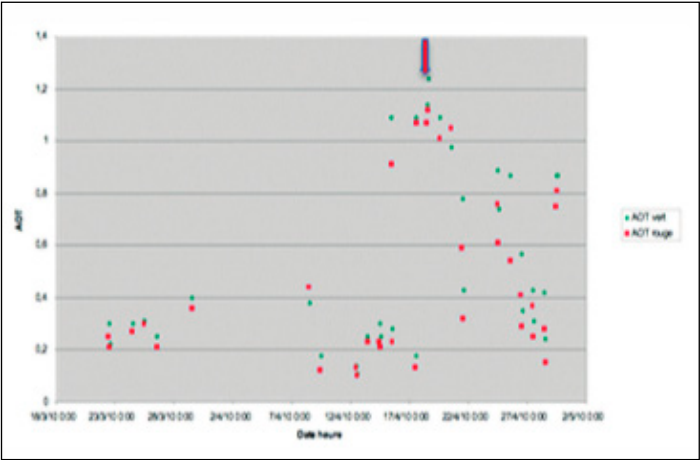
Graphique des valeurs de l'AOT au cours de la campagne de mesures
