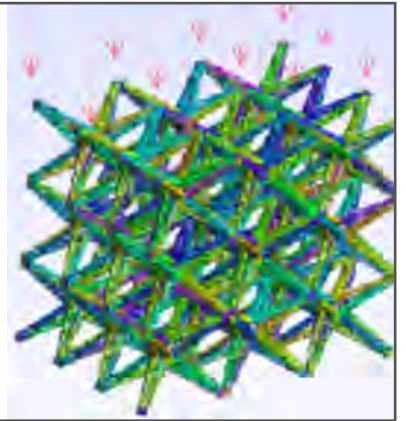
Modélisation EF pour recalibrer une approche analytique d'estimation de la raideur effective (PIMM).
