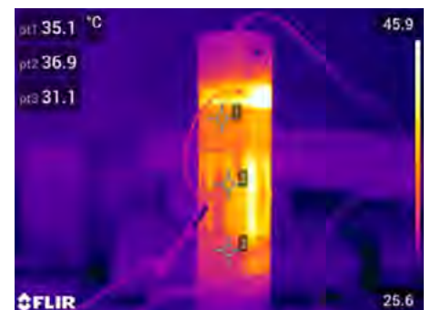
Essai sur un prototype de l'efficacité du graphène comme solution de réchauffeur de lignes d'ergols (Blackleaf).
